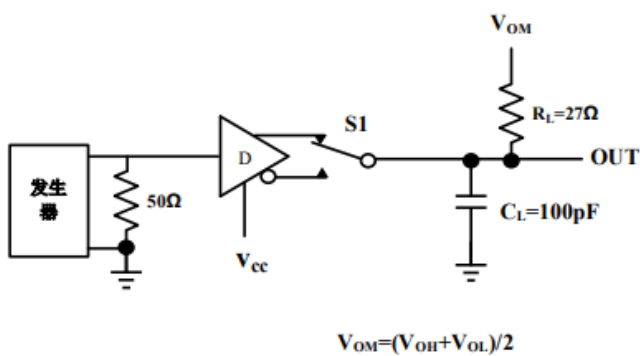
图 4 驱动器传播延迟
